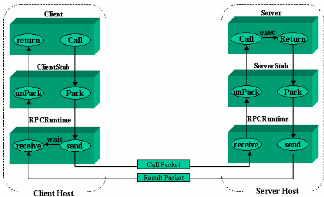
Hình 4.1 Kiến trúc chương trình kiểu RPC
