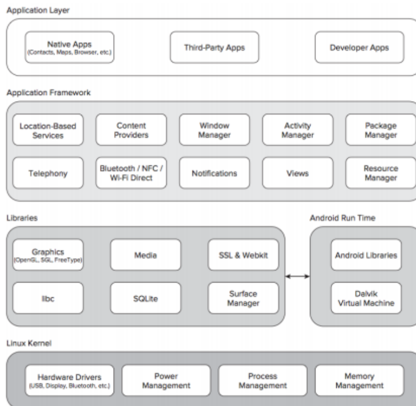
Hình 2.2-1: Các lớp phần mềm trong Android
