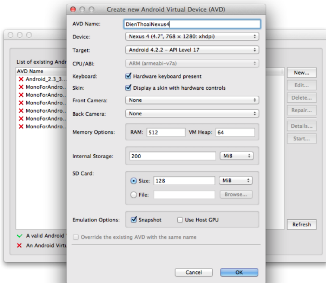
Hình 2.2-6: Tạo thiết bị giả lập Android mới
