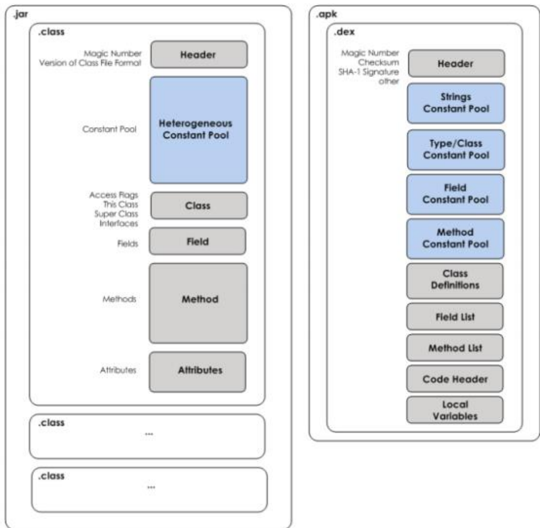
Hình 2.1-6: Cấu trúc Java class file và file thực thi Dalvik
