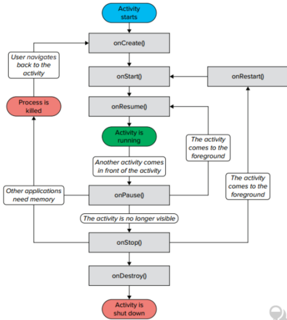
Hình 3.1-1: Vòng đời của một Activity
