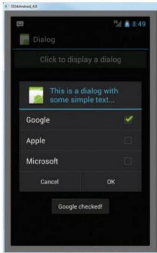
Hình 3.1-2: Hộp thoại
